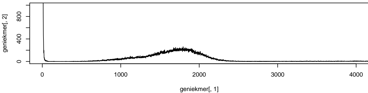
KmerGenie k=23
