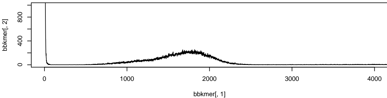
KmerCountExact k=23
